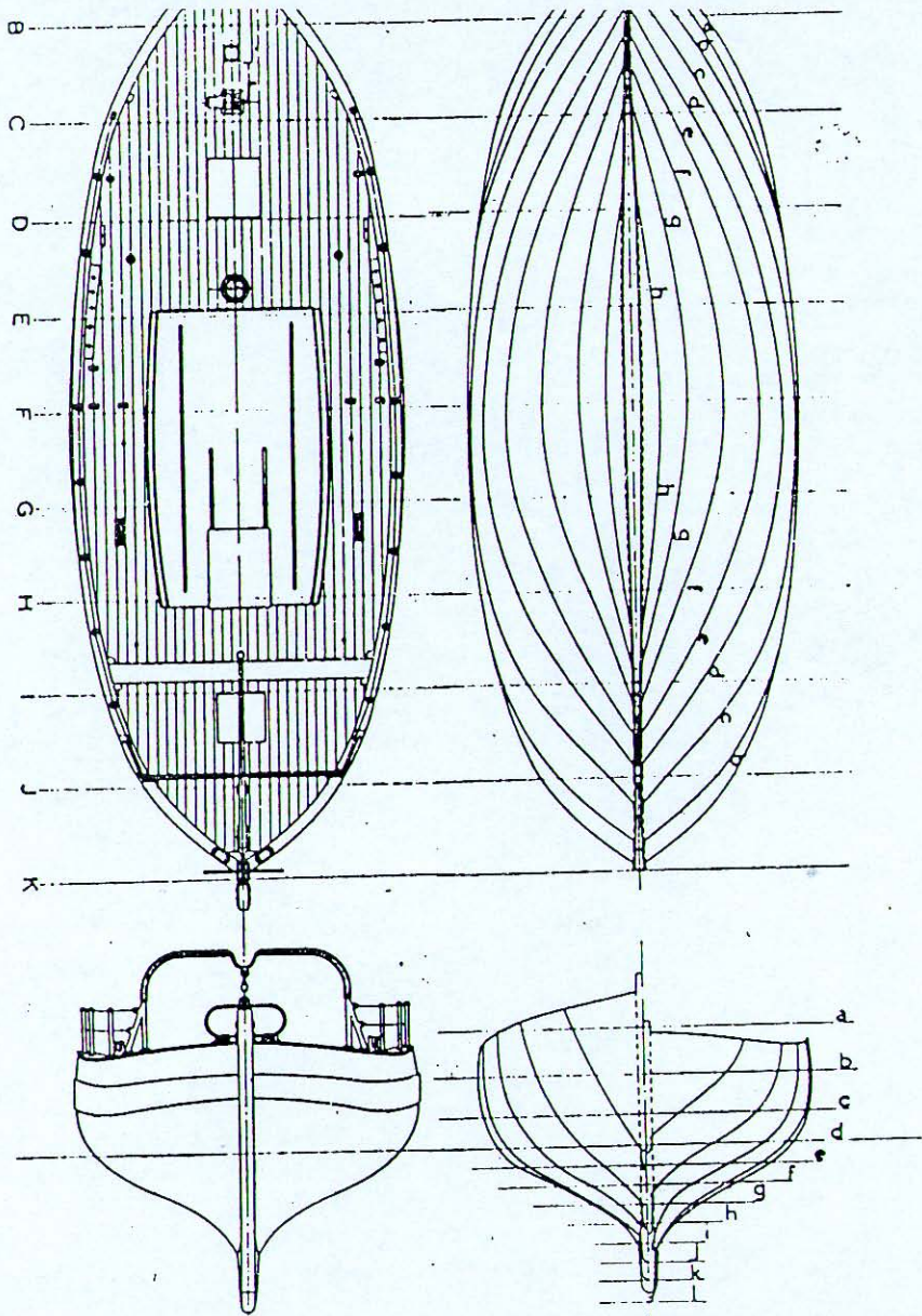
Coupes Verticales
